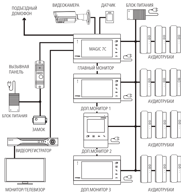
Рис. 9 Функциональная схема системы на базе главного видеодомофона MAGIC 7С
