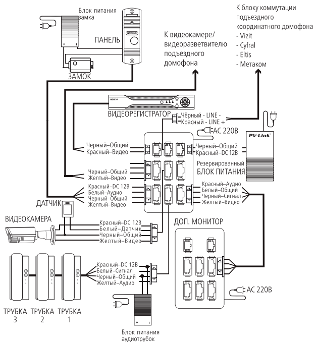
Рис. 11 Схема подключения видеодомофона MAGIC 7C
