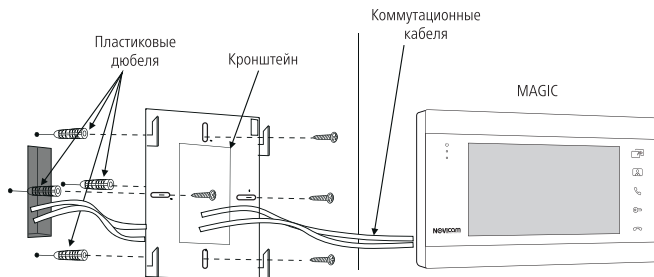
Рис. 6 Монтаж видеодомофона
