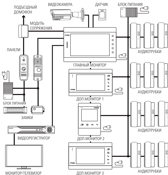
Рис. 8 Функциональная схема системы на базе видеодомофонов MAGIC 4|MAGIC 7|MAGIC 10
