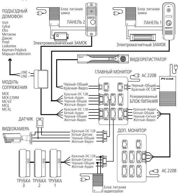
Рис. 10 Схема подключения видеодомофонов MAGIC 4 | MAGIC 7 | MAGIC 10
